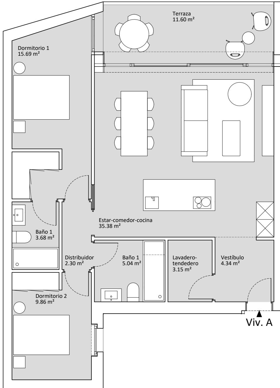
PORTAL 1 PLANTA TIPO Viv. A
